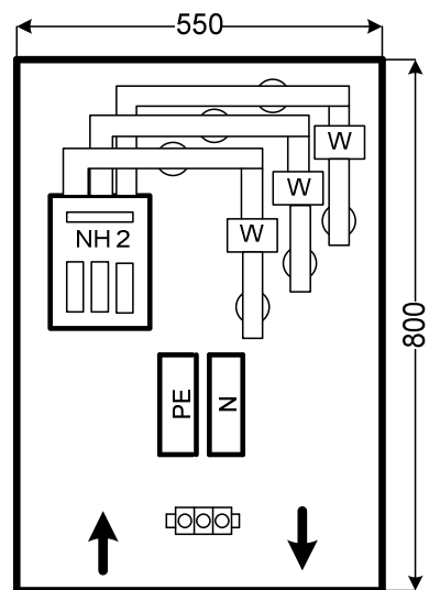
A 2.05 Wandlerschrank 800 x 550 mm (Primärnennstrom max.: 250 A)
